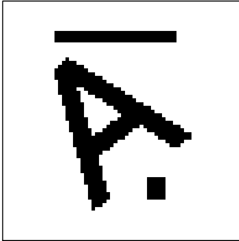
True 0/1
