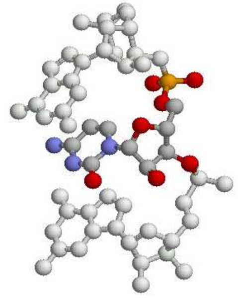
Cytosine
